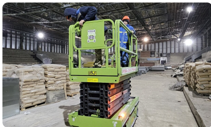
Ножничный подъёмник в цехе
